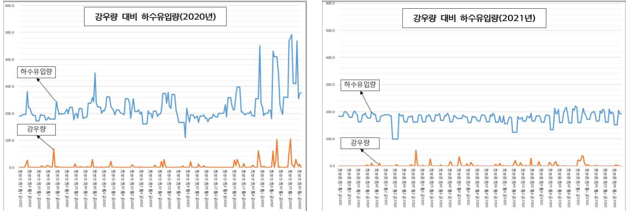
[그림] 연도별 강우량 대비 하수유입량
